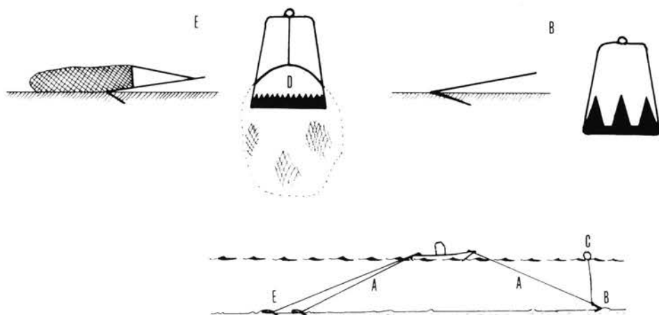
Fig. 16.—Rastros para la pesca de moluscos. A, Garga. B, Gavilán. C, Orinque. D, Peine. E, Rastro
