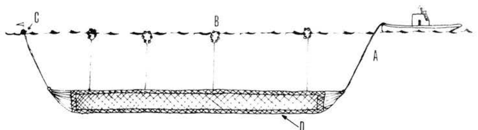
Fig. 5.—Arte de pesca "sardinal". A, Arcera. B, Bornoi. C, Boya, gallo. D, Cadeneta
