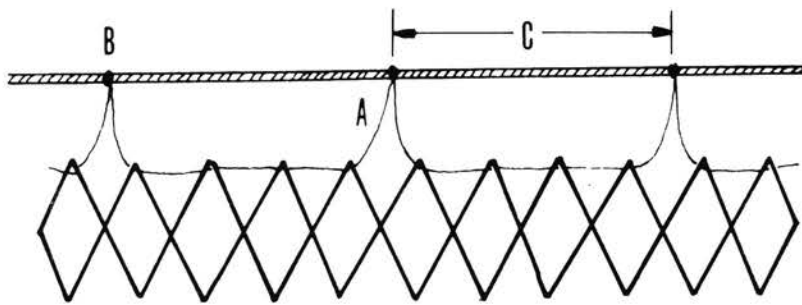
Fig. 1.—Armazón de una red de enmalle y arrastre de playa. A, Armazón. B, Braguerote. C, Abuela o derrame
