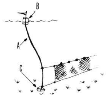
Fig. 3.—Arte de enmalle calado. A, Beta. B, Baliza, boya, gallo o cabecera. C, Cabeceros, hierro, potala o pedrala
