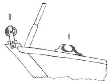
Fig. 4.—Detalle de la proa de una embarcación. A, Biton. B, Garrucha
