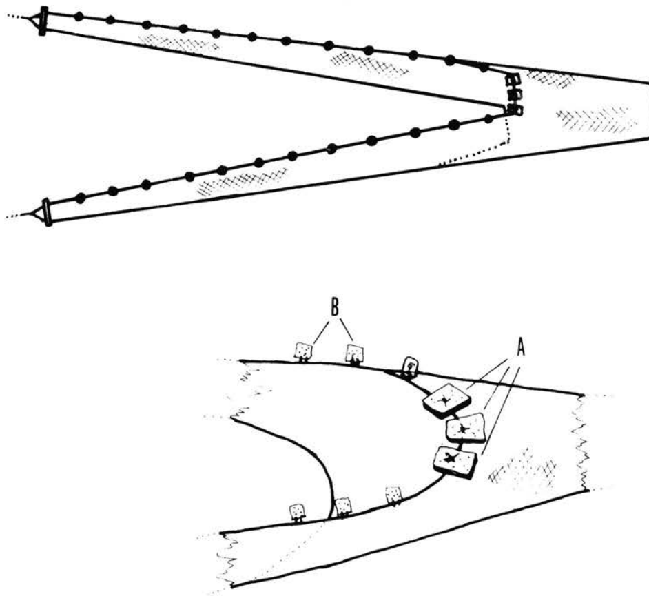
Fig. 17.—Forma y detalle del arte de pesca denominado "jábega". A, Maesa. B, Panda, corchos
