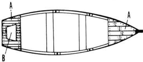
Fig. 9.—Vista superior de una embarcación tipo "chalana", o "chanca". A, Cuarteles. B, Gusín
